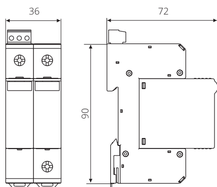
ISPRO C(R) 80/xxx (1+1)
