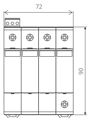
ISPRO C(R) 160/xxx (3+1)
