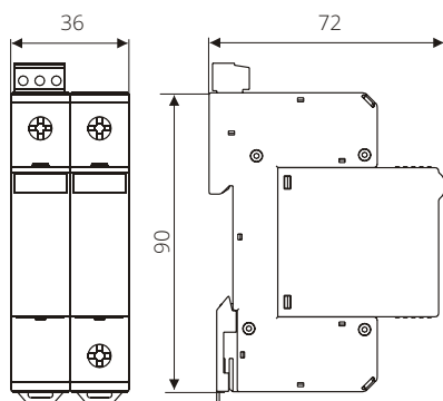
PV ISPRO C(R) 40/550
